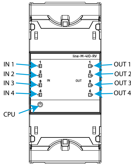
Figura 23: LEDs: line-M-4IO-RV.
