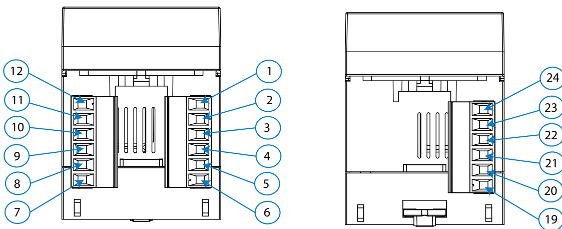
Figura 13: Bornes del line-M-4IO-T: Superior - Inferior.
