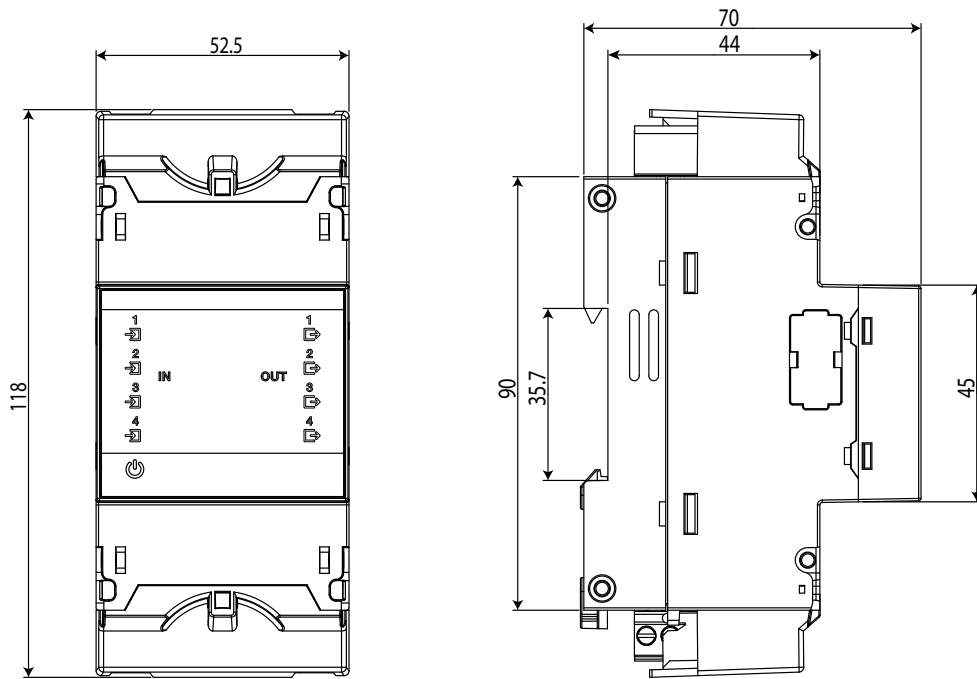
Figura 12: Dimensiones line-M.
