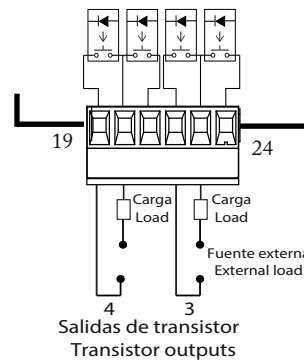
Figura 14: Esquemas de conexión line-M-4IO-T.
