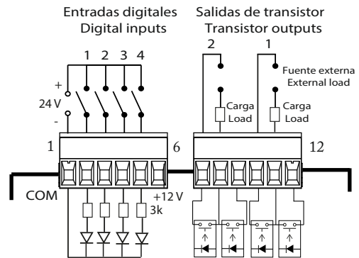
Activación de las Entradas digitales con una fuente externa (+24 V)
