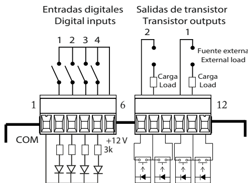
Activación de las Entradas digitales con la fuente interna del equipo (+12 V)
